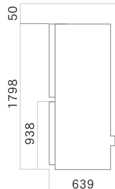
据付スペース (単位mm)
